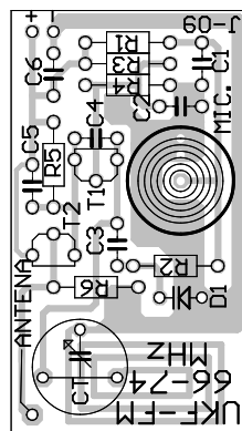
Rysunek płytki
