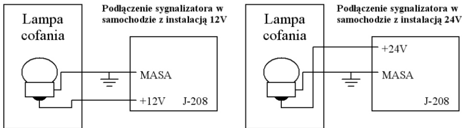
Sposób podłączenia
