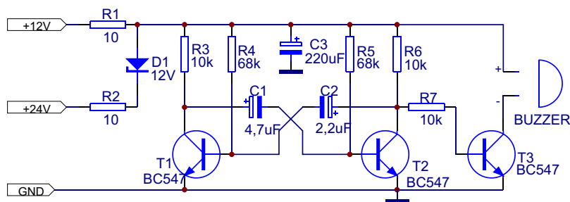
Schemat ideowy
